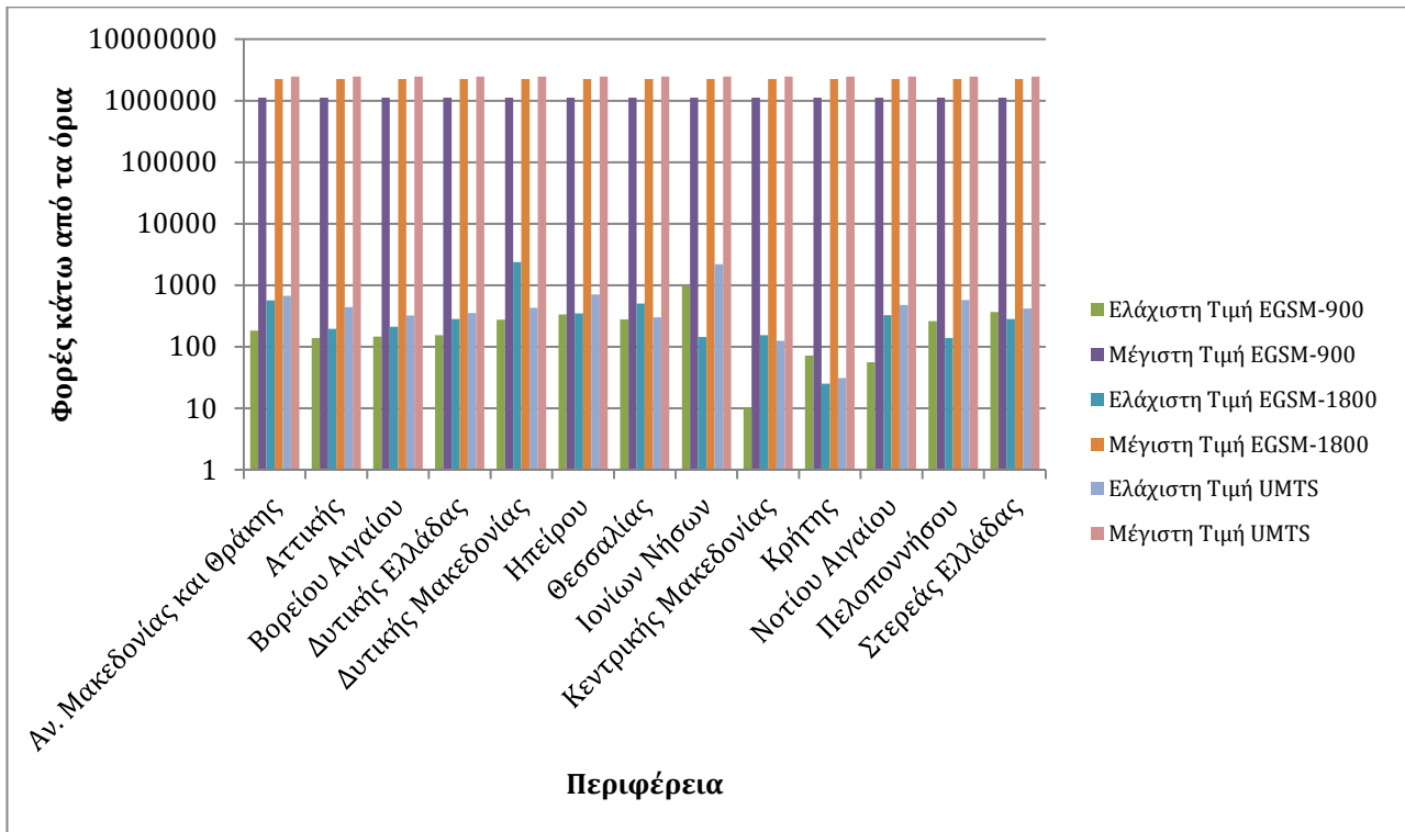
Διάγραμμα 4: Φορές κάτω από τα όρια των τιμών έντασης ηλεκτρικού πεδίου ανά Περιφέρεια (τιμές υποπεριοχών συχνοτήτων GSM-900, EGSM-1800, UMTS-2100)
