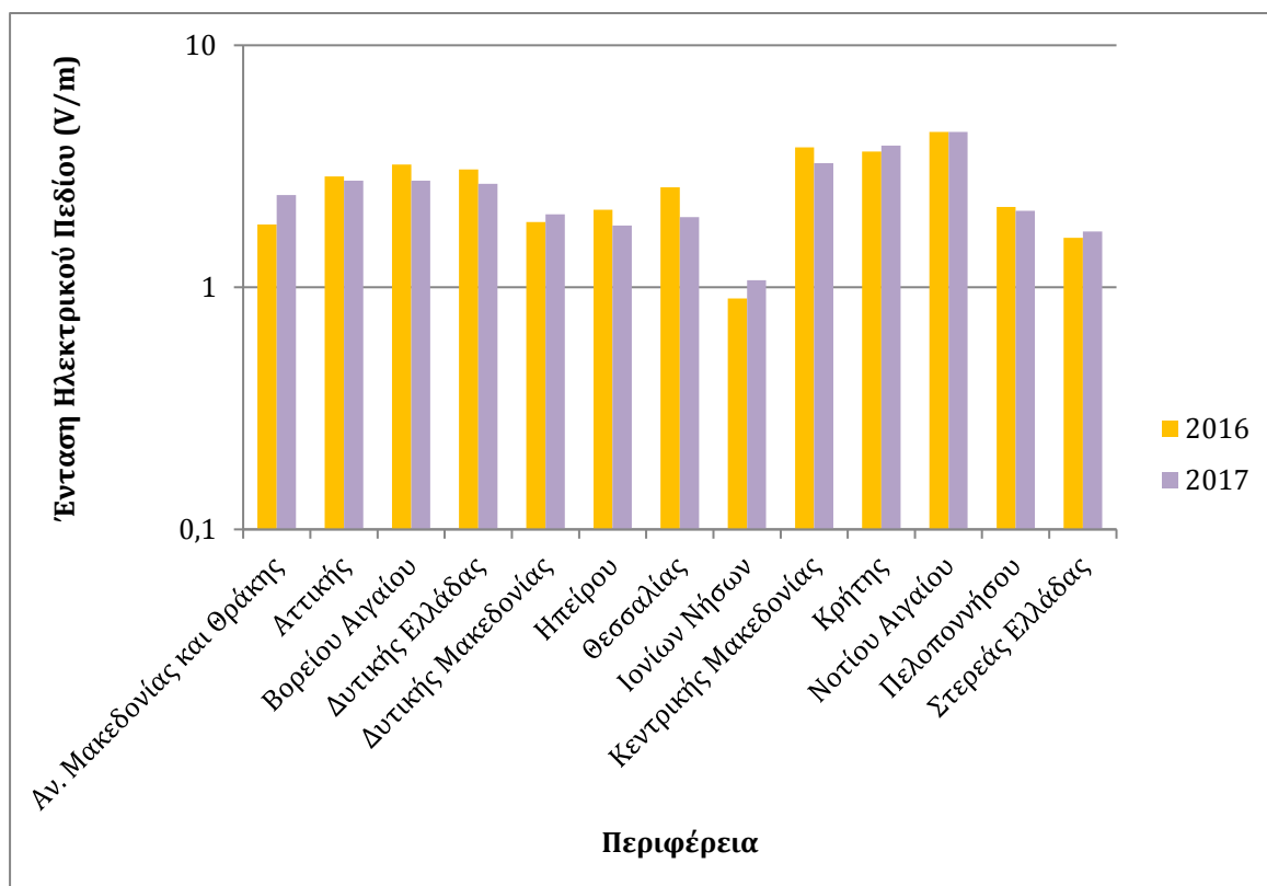
Διάγραμμα 7: Μέγιστες ημερήσιες μέσες τιμές έντασης ηλεκτρικού πεδίου (V/m) ανά Περιφέρεια (Υποπεριοχή συχνοτήτων EGSM-1800) για τα έτη 2016 & 2017
