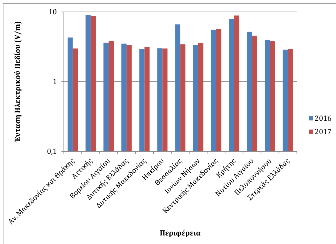
Διάγραμμα 5: Μέγιστες ημερήσιες μέσες τιμές έντασης ηλεκτρικού πεδίου (V/m) ανά Περιφέρεια (Ευρυζωνικές τιμές 100 kHz - 7 GHz) για τα έτη 2016 & 2017
