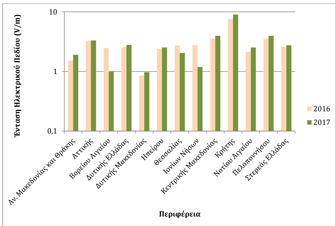
Διάγραμμα 7: Μέγιστες ημερήσιες μέσες τιμές έντασης ηλεκτρικού πεδίου (V/m) ανά Περιφέρεια (Υποπεριοχή συχνοτήτων EGSM-1800) για τα έτη 2016 & 2017
