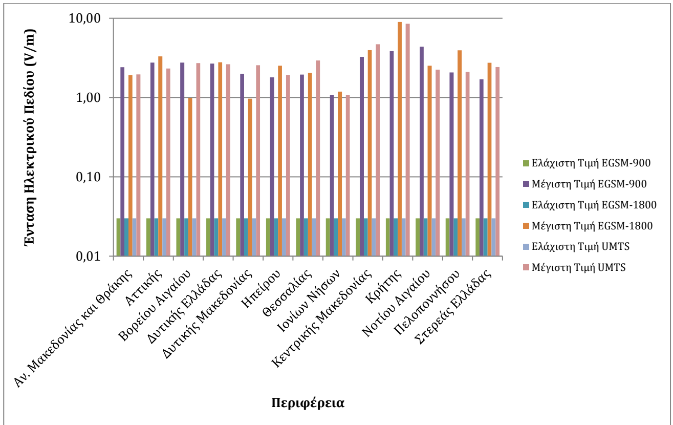
Διάγραμμα 2: Εύρος μέσων τιμών έντασης ηλεκτρικού πεδίου (V/m) ανά Περιφέρεια (τιμές υποπεριοχών συχνοτήτων GSM-900, EGSM-1800, UMTS-2100)
