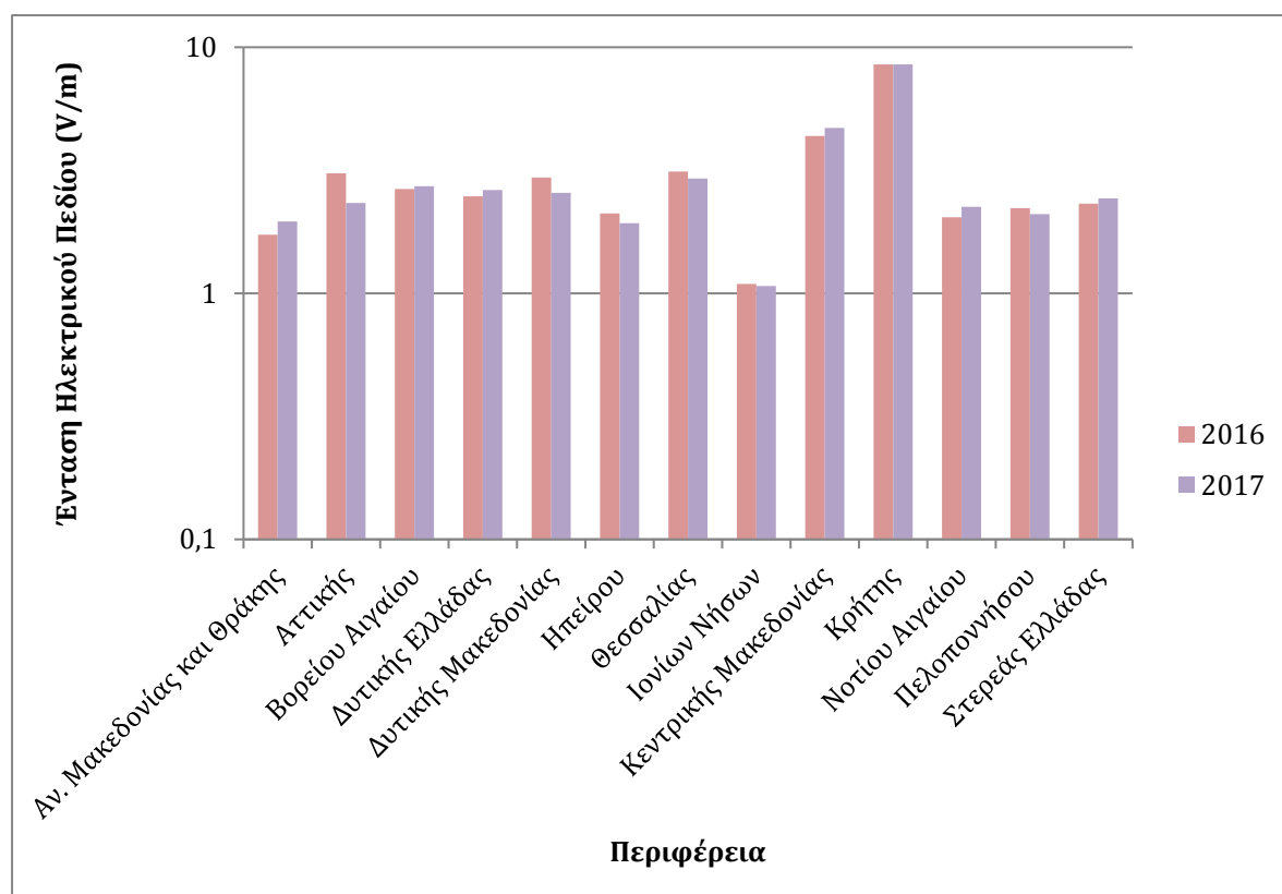
Διάγραμμα 8: Μέγιστες ημερήσιες μέσες τιμές έντασης ηλεκτρικού πεδίου (V/m) ανά Περιφέρεια (Υποπεριοχή συχνοτήτων UMTS) για τα έτη 2016 & 2017
