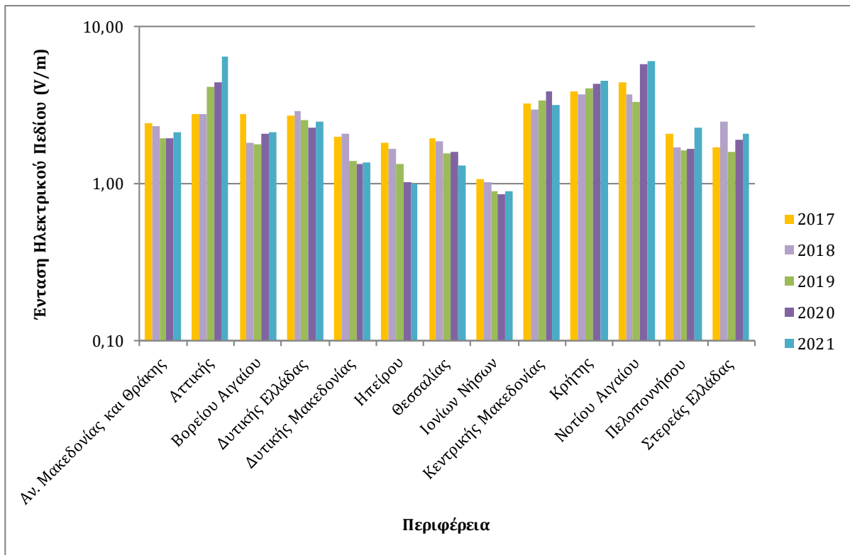
Διάγραμμα 7: Μέγιστες ημερήσιες μέσες τιμές έντασης ηλεκτρικού πεδίου (V/m) ανά Περιφέρεια (υποπεριοχή συχνοτήτων EGSM-1800) για τα έτη 2017, 2018, 2019, 2020 & 2021
