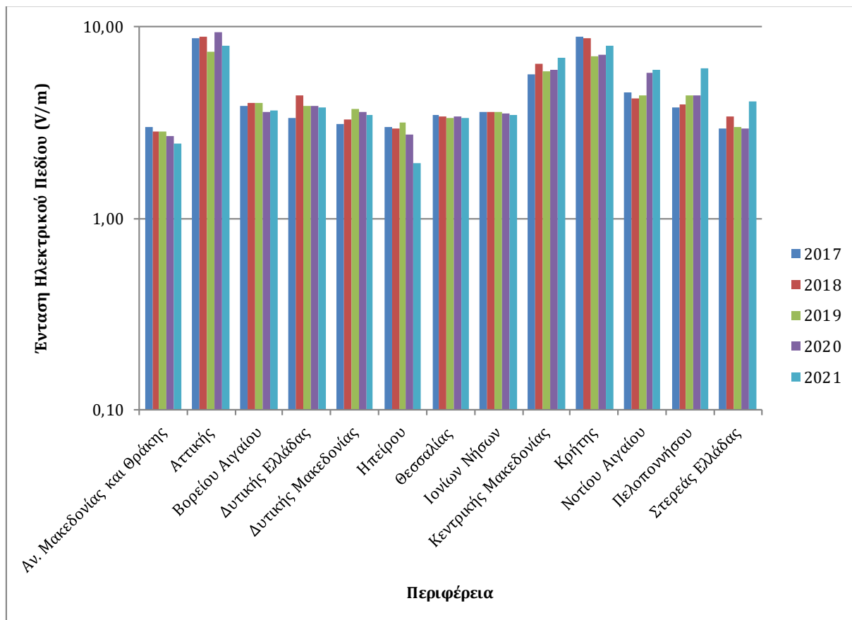
Διάγραμμα 5: Μέγιστες ημερήσιες μέσες τιμές έντασης ηλεκτρικού πεδίου (V/m) ανά Περιφέρεια (Ευρυζωνικές τιμές 100 kHz - 7 GHz) για τα έτη 2017, 2018, 2019, 2020 & 2021
