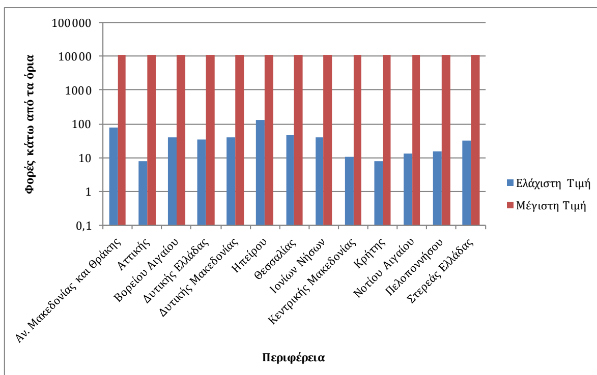
Διάγραμμα 3: «Φορές κάτω από τα όρια» των τιμών έντασης ηλεκτρικού πεδίου ανά Περιφέρεια (ευρυζωνικές τιμές 100 kHz - 7 GHz)
