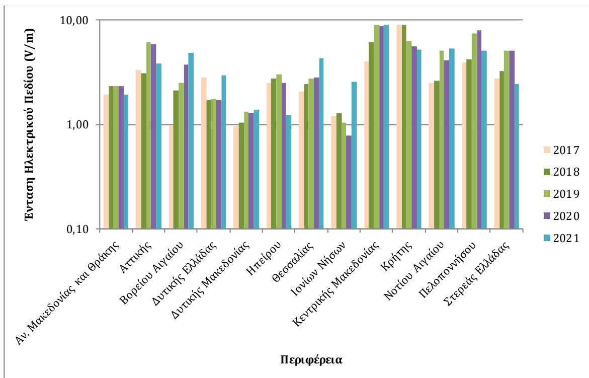
Διάγραμμα 8: Μέγιστες ημερήσιες μέσες τιμές έντασης ηλεκτρικού πεδίου (V/m) ανά Περιφέρεια (υποπεριοχή συχνοτήτων UMTS) για τα έτη 2017, 2018, 2019, 2020 & 2021
