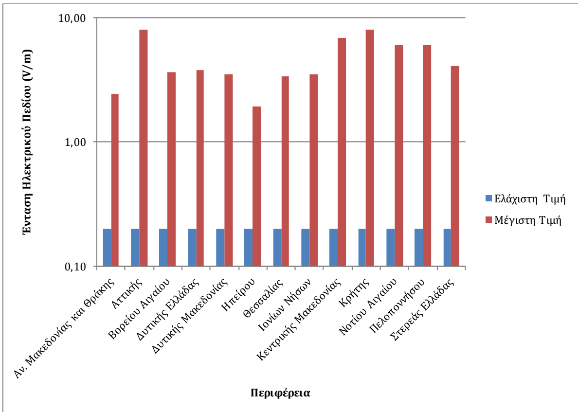
Διάγραμμα 1: Εύρος μέσων τιμών έντασης ηλεκτρικού πεδίου (V/m) ανά Περιφέρεια (Ευρυζωνικές τιμές 100 kHz - 7 GHz)
