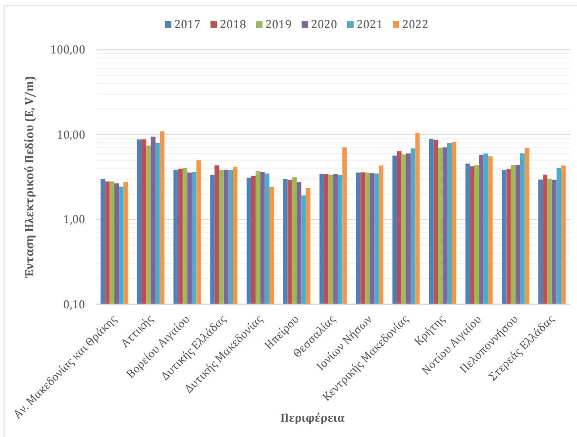
Διάγραμμα 5: Μέγιστες ημερήσιες μέσες τιμές έντασης ηλεκτρικού πεδίου (V/m) ανά Περιφέρεια (Ευρυζωνικές τιμές 100 kHz - 7 GHz) για τα έτη 2017-2022
