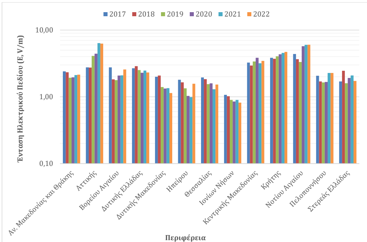
Διάγραμμα 6: Μέγιστες ημερήσιες μέσες τιμές έντασης ηλεκτρικού πεδίου (V/m) ανά Περιφέρεια (υποπεριοχή συχνοτήτων GSM-900) για τα έτη 2017- 2022
