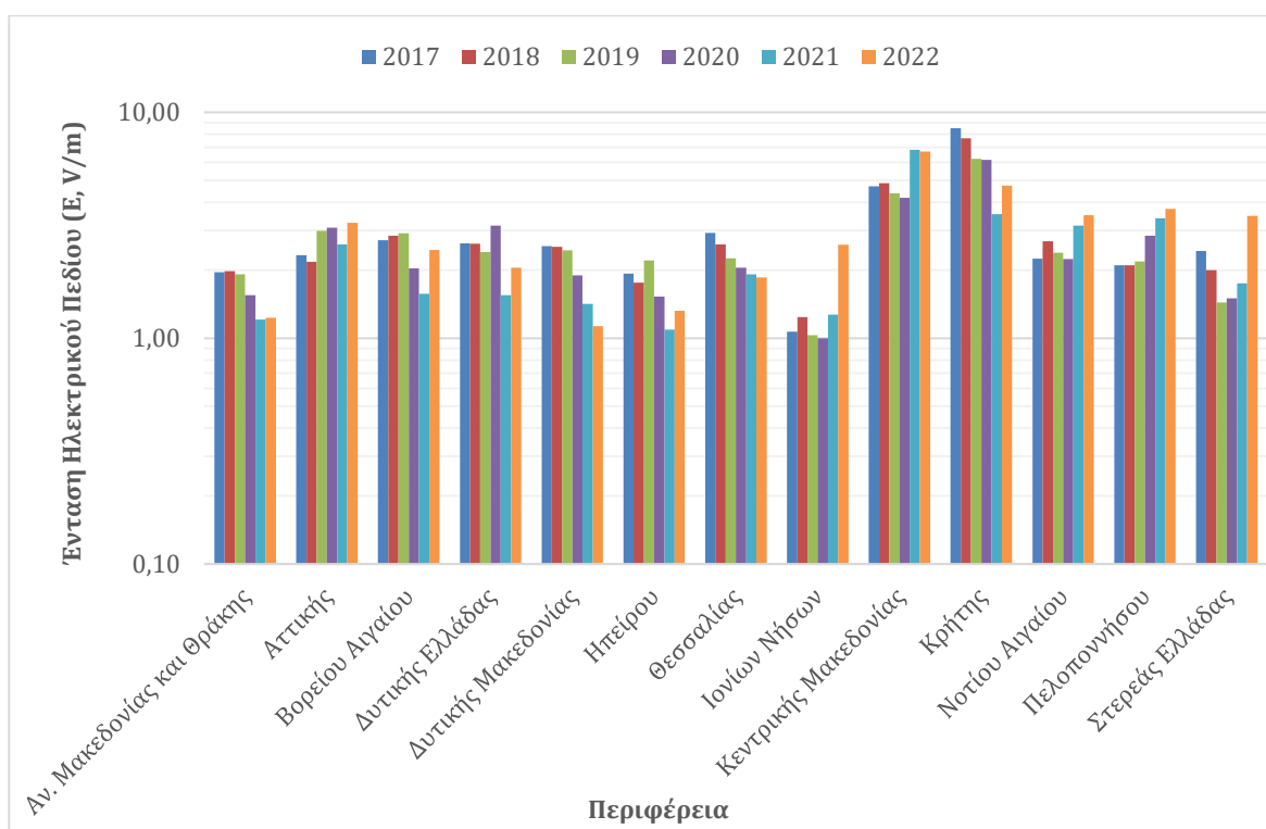
Διάγραμμα 8: Μέγιστες ημερήσιες μέσες τιμές έντασης ηλεκτρικού πεδίου (V/m) ανά Περιφέρεια (υποπεριοχή συχνοτήτων UMTS) για τα έτη 2017- 2022
