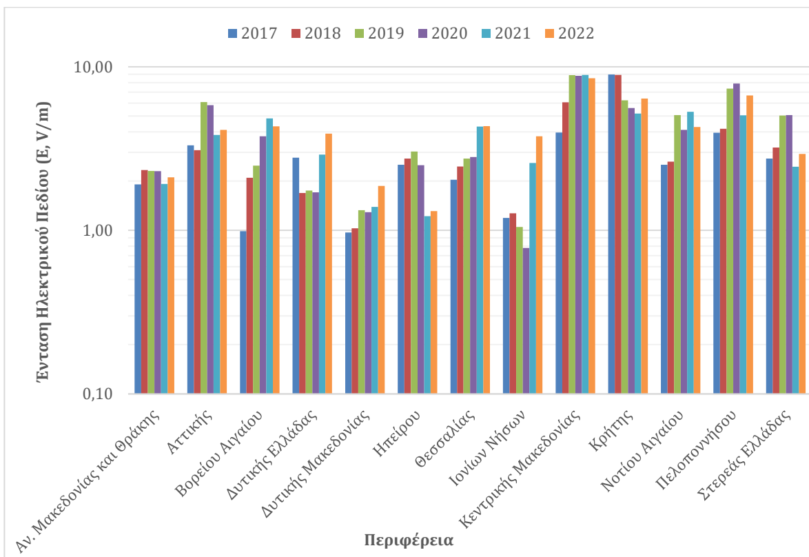
Διάγραμμα 7: Μέγιστες ημερήσιες μέσες τιμές έντασης ηλεκτρικού πεδίου (V/m) ανά Περιφέρεια (υποπεριοχή συχνοτήτων EGSM-1800) για τα έτη 2017- 2022
